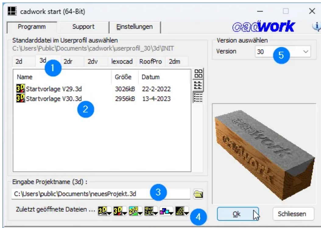
Reiter Programm im cadwork Start
